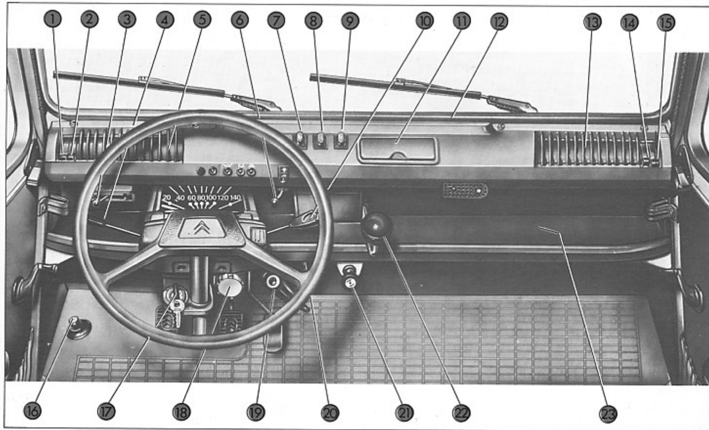
Fig. 7 - Posto di guida : comandi e accessori
