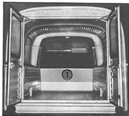
Fig. 24 - 1 - Paratia di separazione dietro i sedili anteriori
