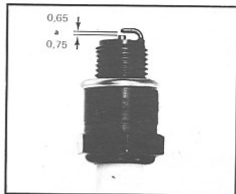
Fig. 43 - Candela Distanza degli elettrodi
